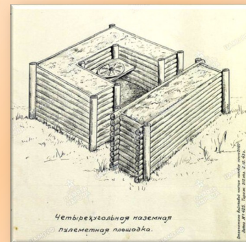
Четырёхугольная наземная пулеметная площадка
